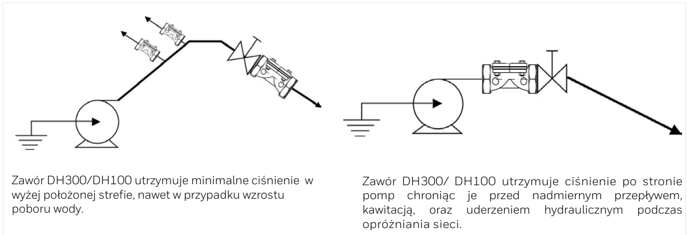
Rys. 1 Standardowy przykład montażu zaworu pierwszeństwa
